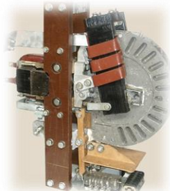
Электропневматический контактор БК-78Т
